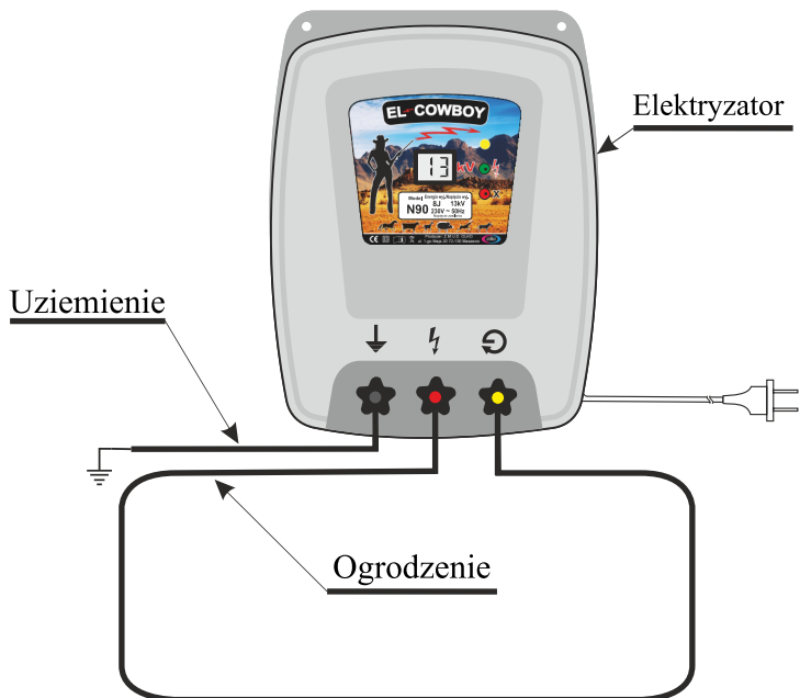
Rys. 4 Kontrola elektryczna ogrodzenia.
