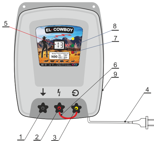
Rys.1 Elektryzator ogrodzenia EL-COWBOY N90
