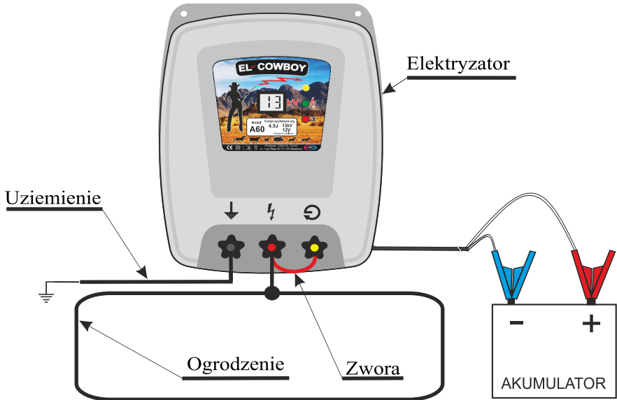
Rys. 2 Brak kontroli elektrycznej ogrodzenia.
