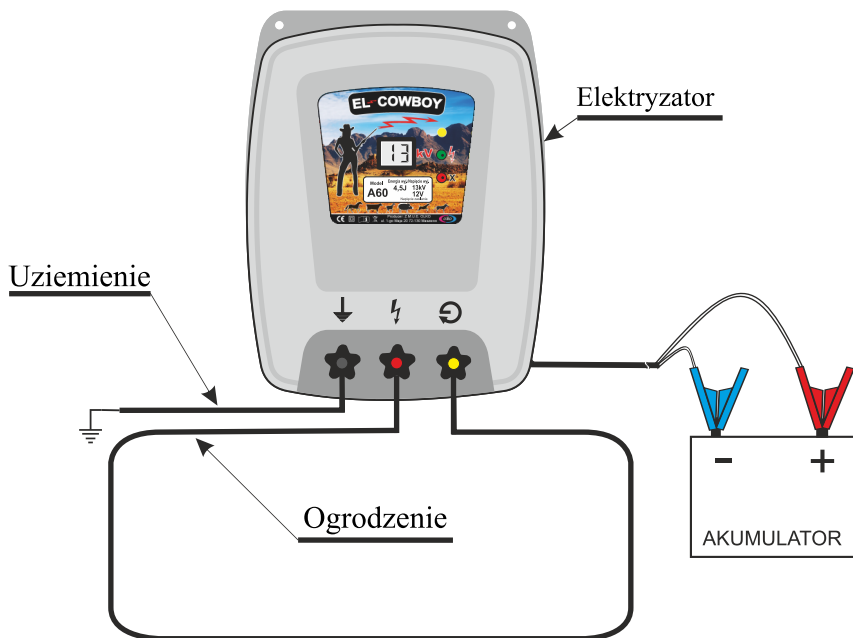
Rys. 4 Kontrola elektryczna ogrodzenia.
