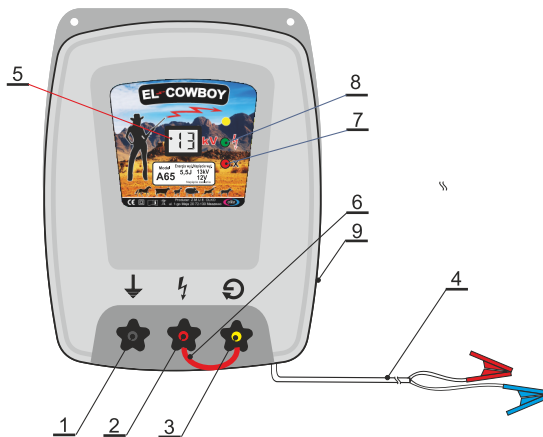
Rys.1 Elektryzator ogrodzenia EL-COWBOY A65
